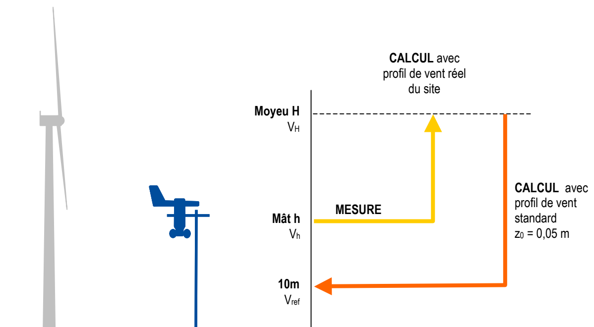
Figure 48 - Principe du calcul de la vitesse de référence à 10 m (source : Acouphen environnement)
