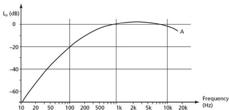
Courbe de pondération A en fonction de la fréquence
