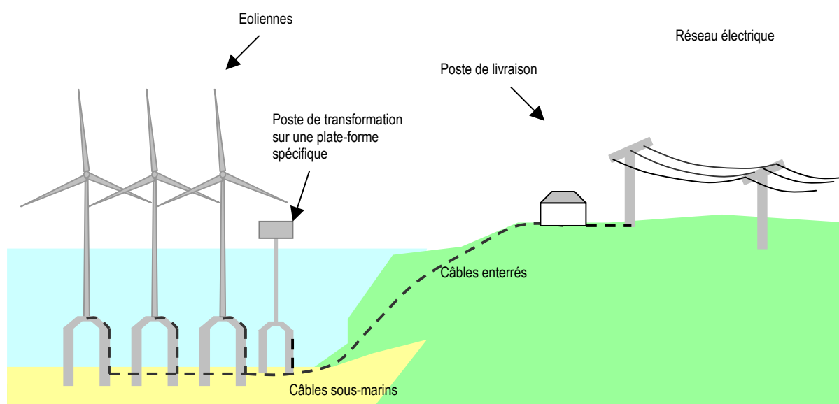
Figure 4 - Schéma d'implantation d'un projet éolien en mer (rapports d'échelle non représentatifs)
