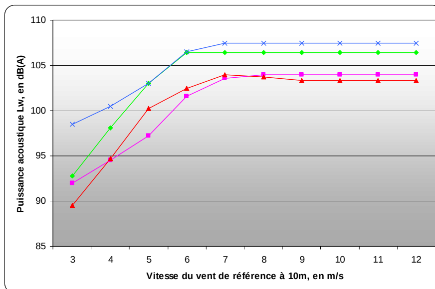
Figure 50 - Exemple d'évolution de la puissance acoustique en fonction de la vitesse du vent (source : Acouphen environnement )
