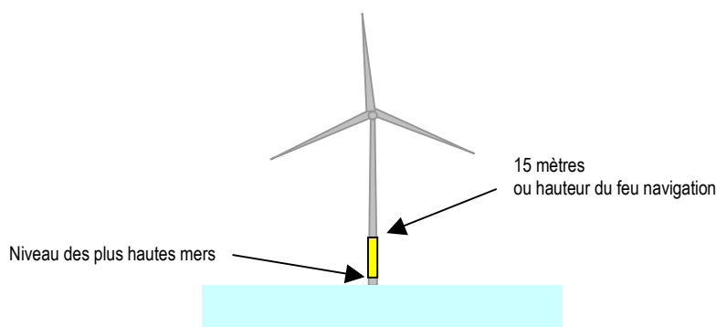
Figure 57 - Signalisation maritime d'une éolienne
